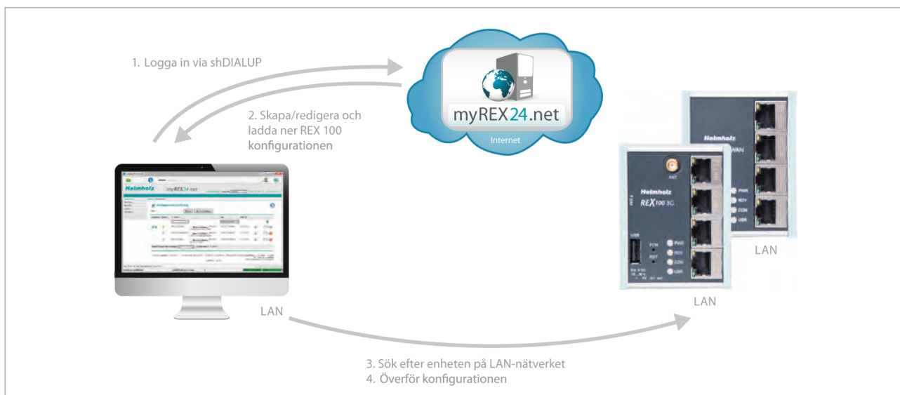
Variant c). Konfiguration via LAN nätverket
