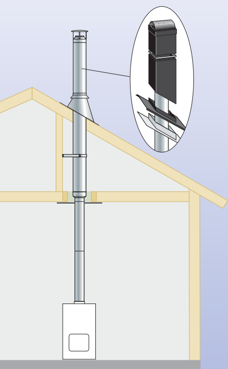
DW ALKON Modulskorsten i syrafast, rostfritt stål, schaktfritt utförande
