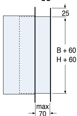
Montage i schaktvägg
