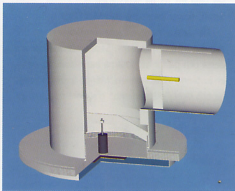
LindinVents aktiva tilluftsdon IDCC.
